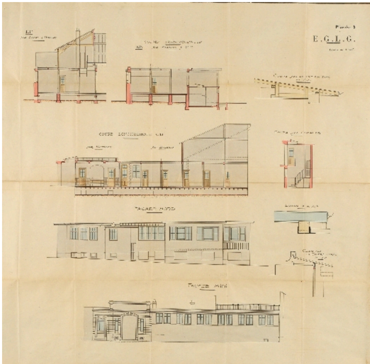
Elévation et coupe des bureaux 1920-1930
