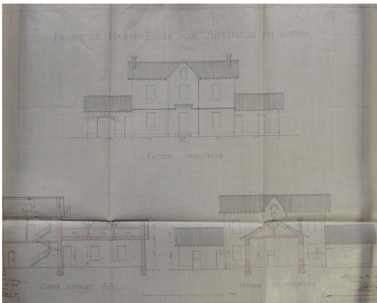
Projet de mairie-école pour Ambérieux-en-Dombes : élévations, 1876 (AD Ain. 2 O 52).
