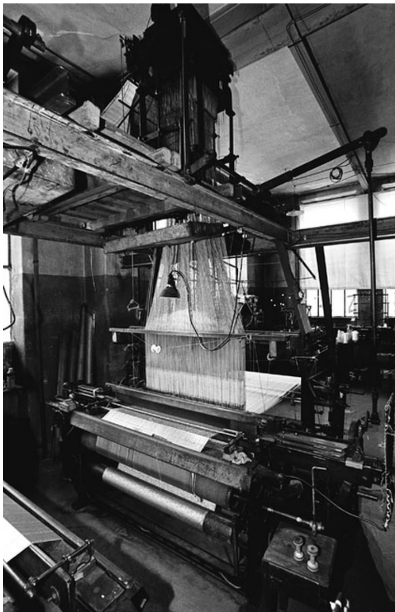
Vue arrière du métier n° 21
