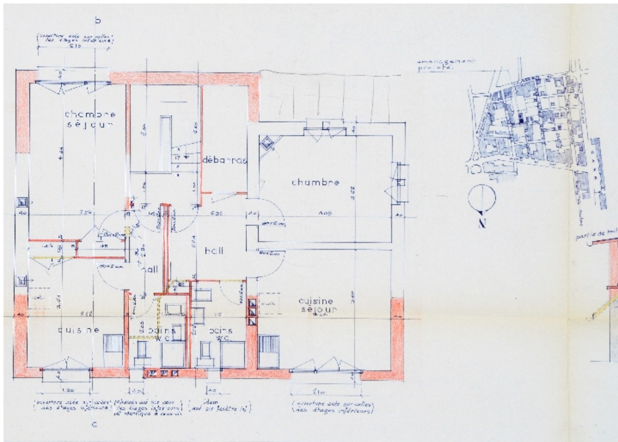
Aménagement de l'étage de combles : plan
