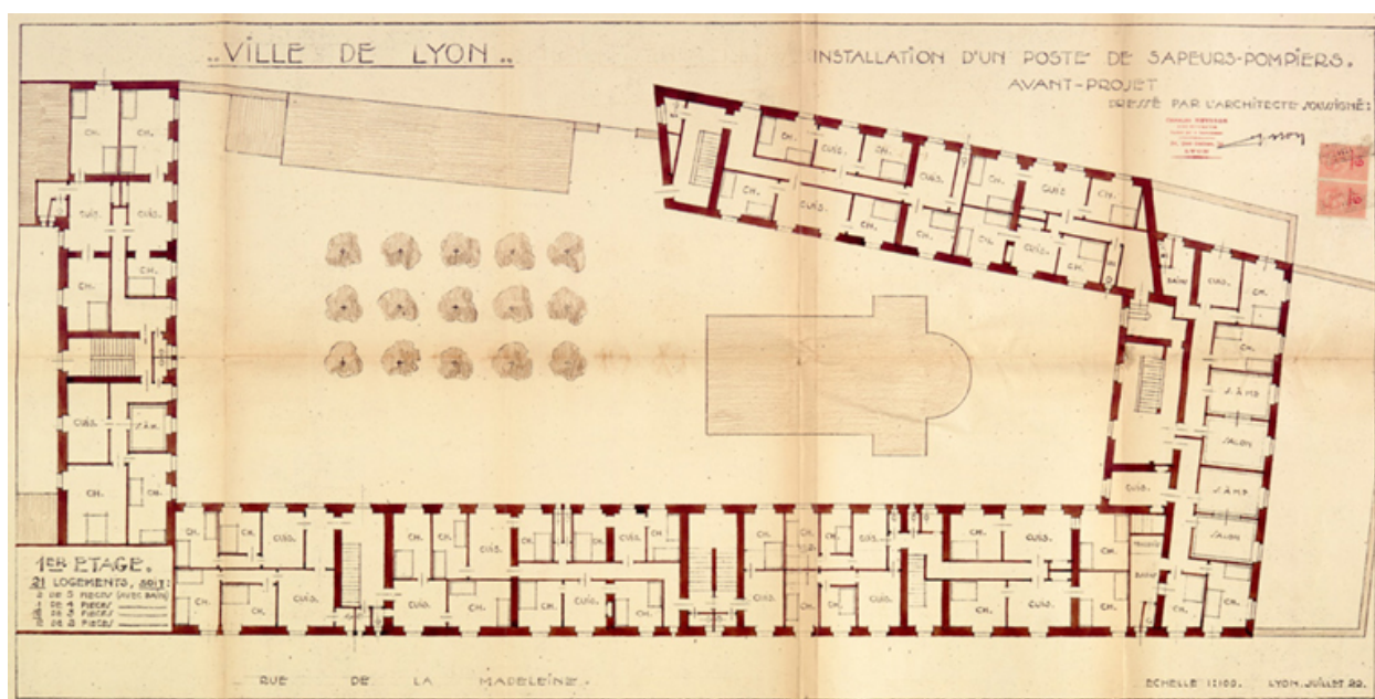
Installation d'un poste de sapeurs-pompiers. Avant-projet, par Charles Meysson, 22 juillet [1922]. Plan du 1er étage. 1 : 100 (AC Lyon. 0470 WP 026)
