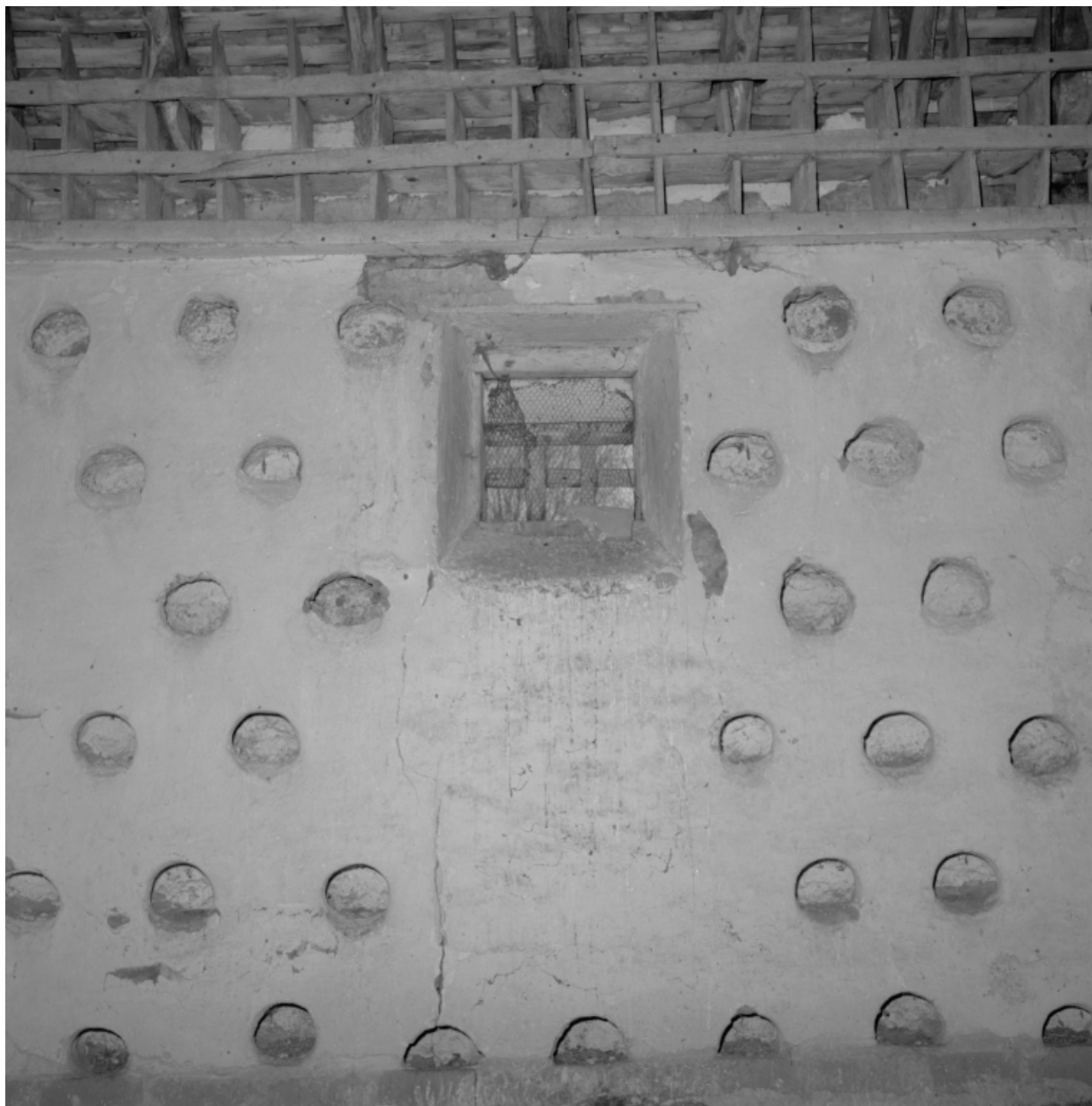
Vue intérieure partielle de la charpente et du mur de surcroît aménagé de boulins.
