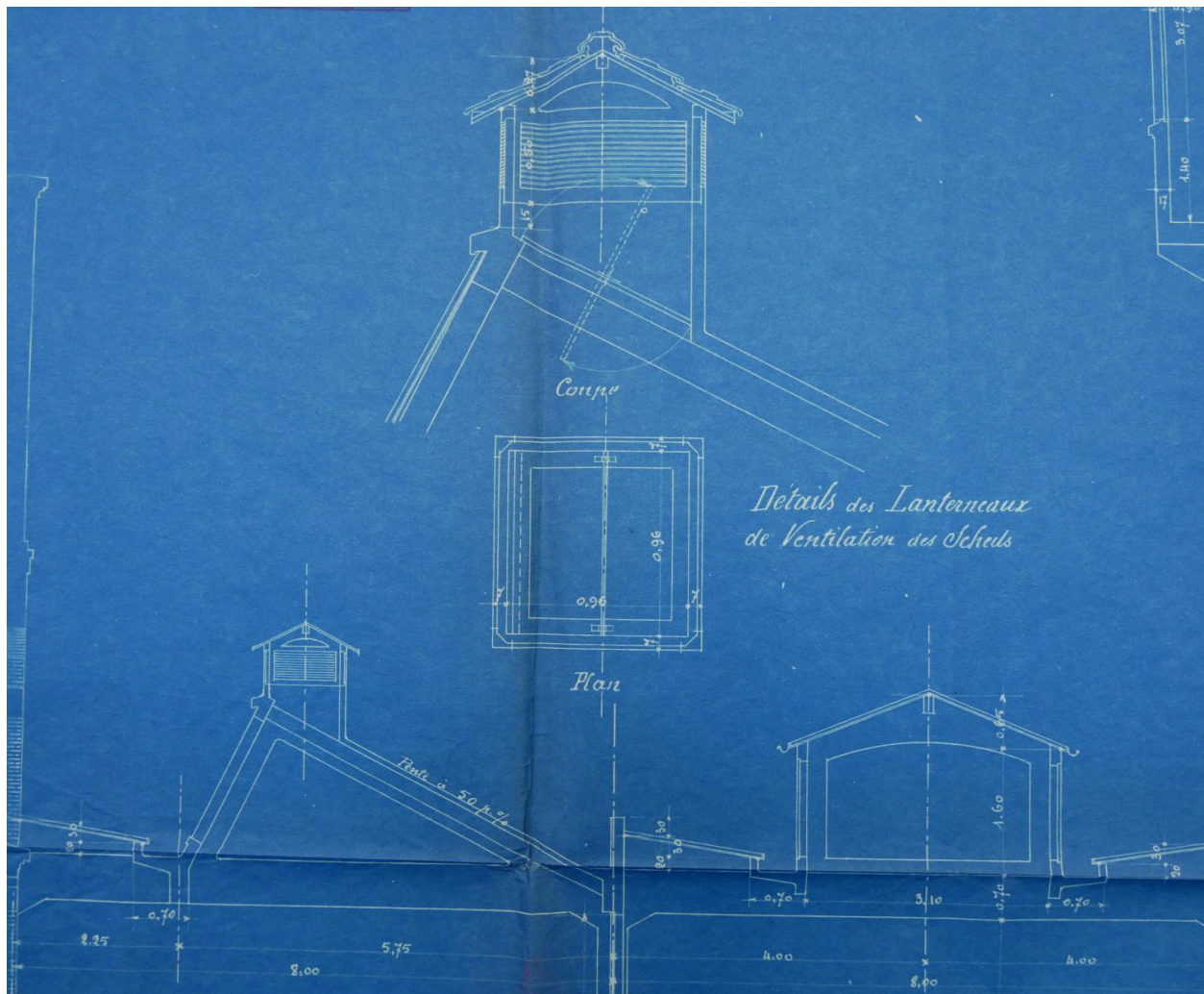
Détail plan usine Seguin 1917 : shed et aérateur (ACL 314W/581)
