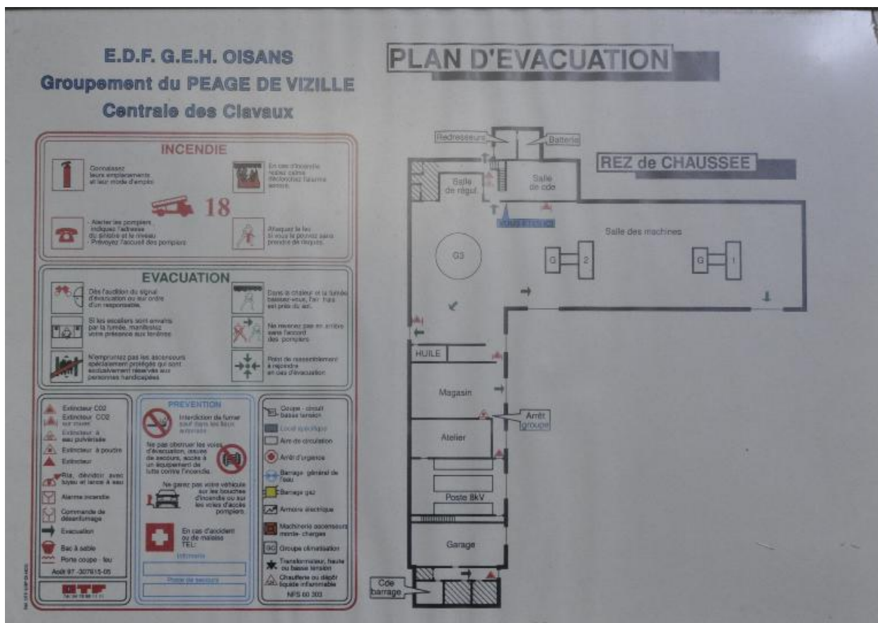
Plan du rez-de-chaussée de la centrale
