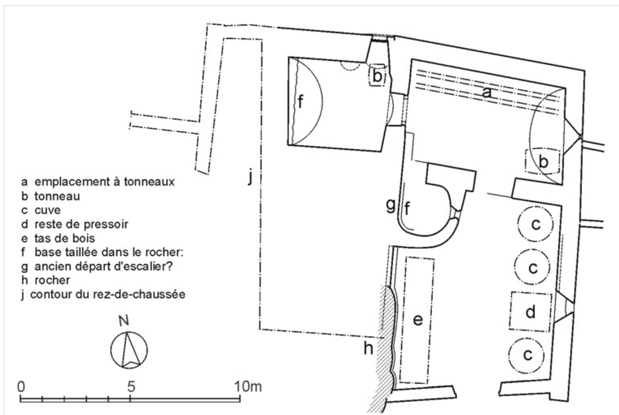
Plan de l'étage de soubassement du bâtiment nord-est.
