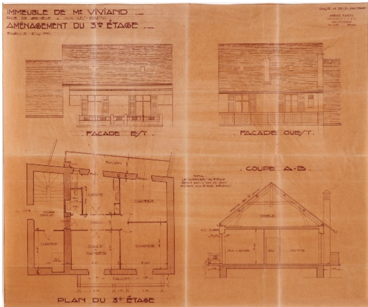
Plan, coupe et élévations du 3e étage
