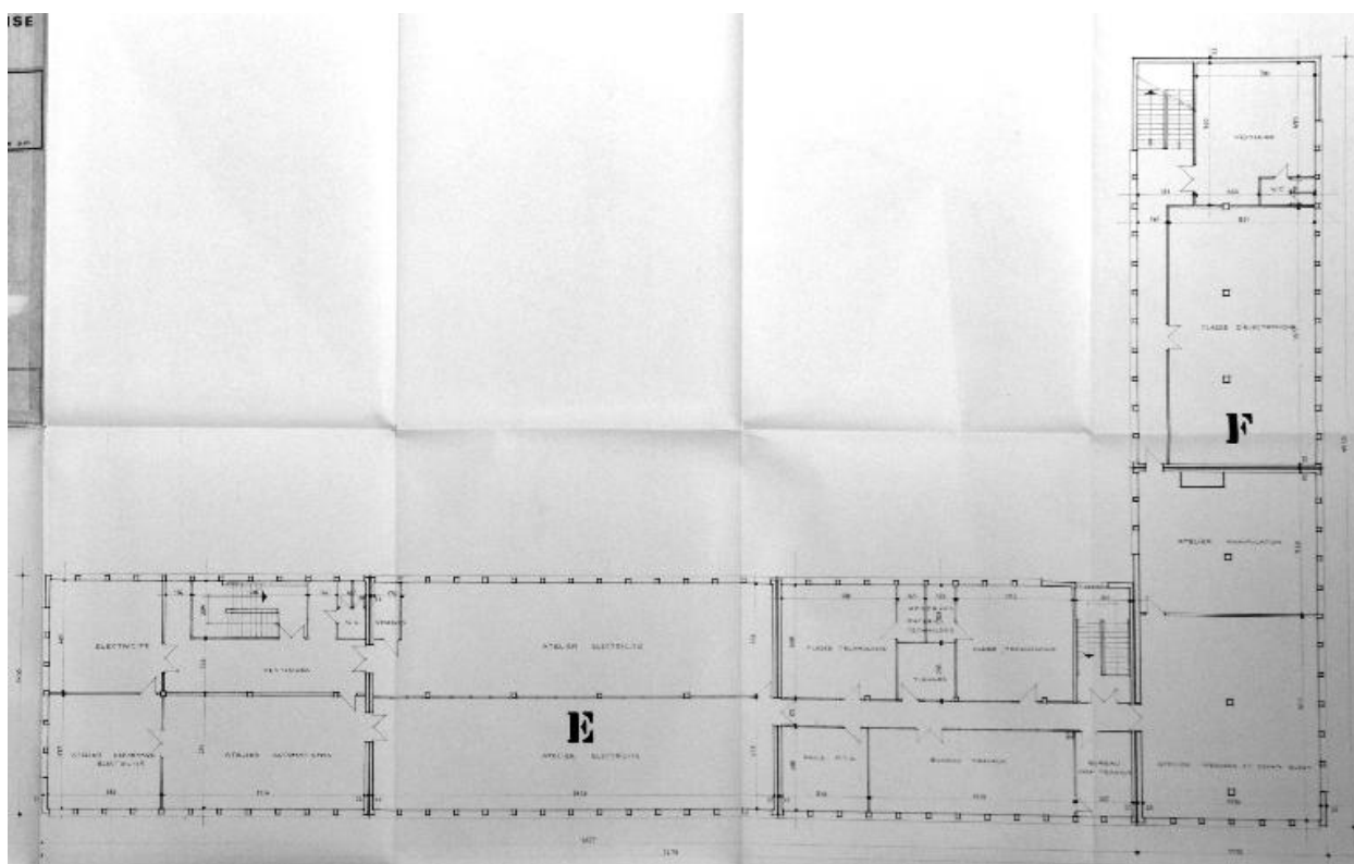
Lycée Technique Nationalisé, Plan bâtiments E et F 1er étage, A. Profit Mai 1974 (AC Ugine, 6 W 106)
