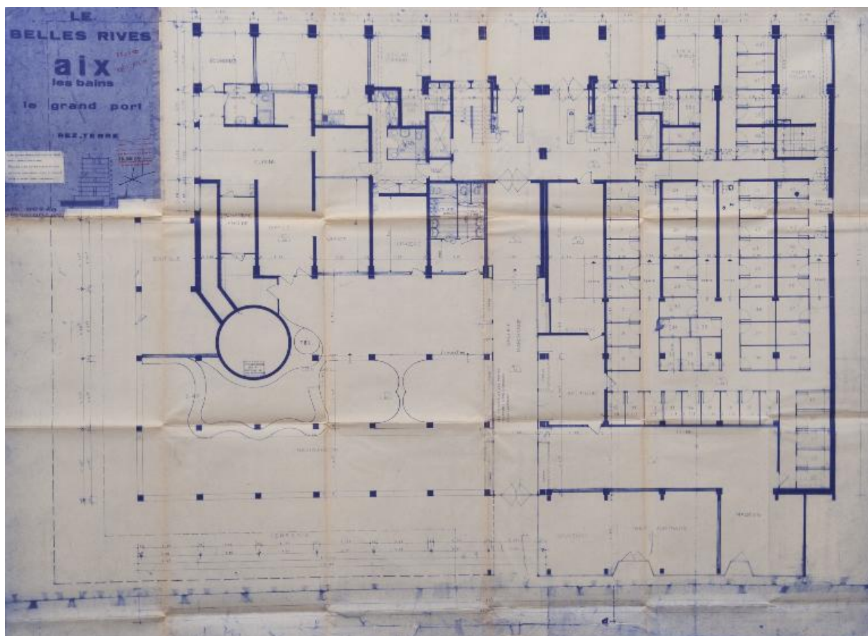
Partie nord, 1968 : plan du rez-de-chaussée
