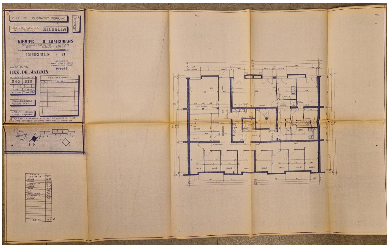
Projet d'un groupe d'immeubles, rues Viviani et du Var (1ère tranche) : plan du rez-de-jardin du bâtiment B, 1976.
