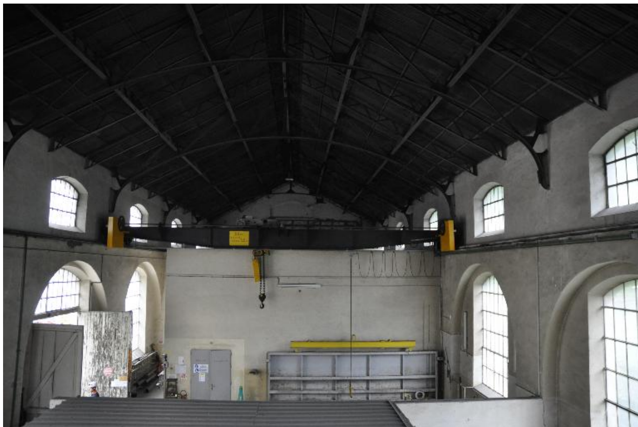
Vue du pont roulant et de la charpente métallique de la salle des machines
