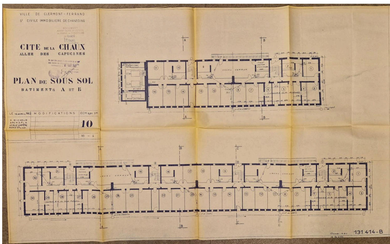
Projet des immeubles "les Capucines" à Lachaux : plan des sous-sols des bâtiments A et B, 1962.
