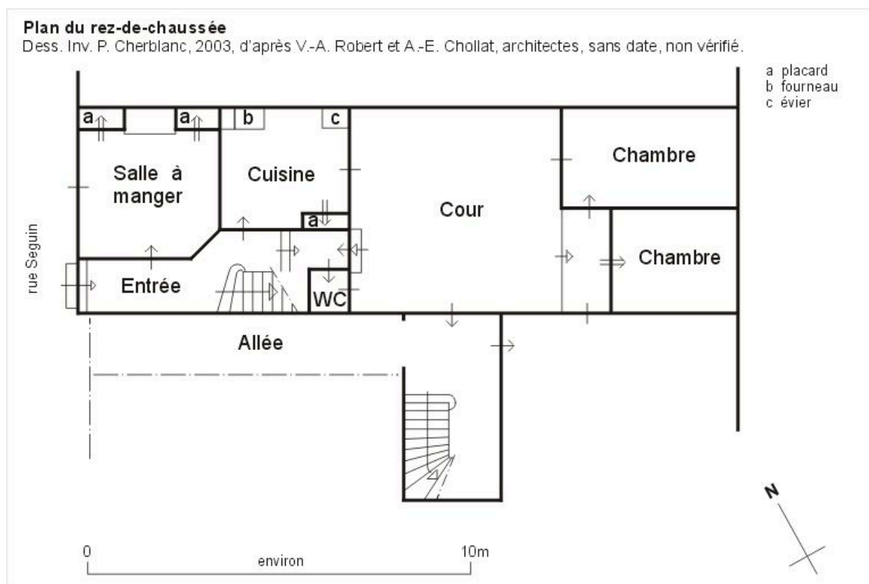
Plan du rez-de-chaussée, d'après V.-A. Robert et A.-E. Chollat
