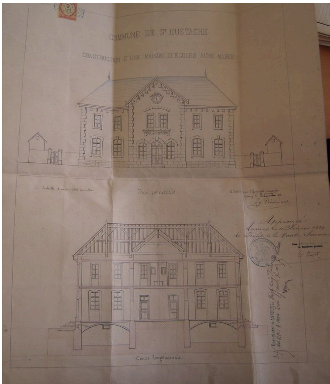
Projet architectural (façade et coupe).
