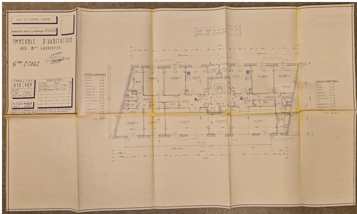
Plan du 6e étage de l'immeuble.
