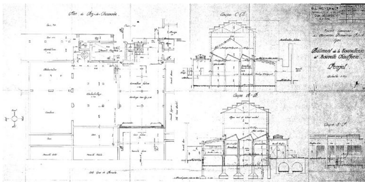
Plan de la tonnellerie / G.L. Meyer et Cie, 1938 (AC Lyon : 1097 WP 097)
