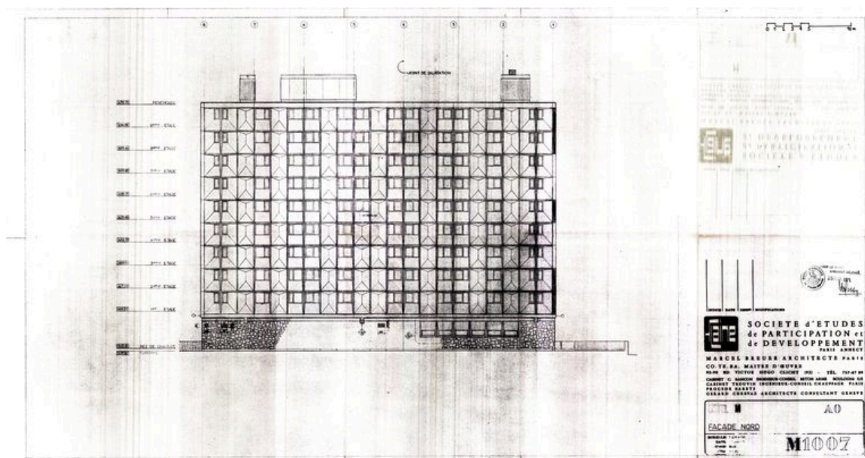
Hôtel M. Élévation nord. Marcel Breuer architecte, 27 janvier 1971 (AC Arâches-la Frasse)
