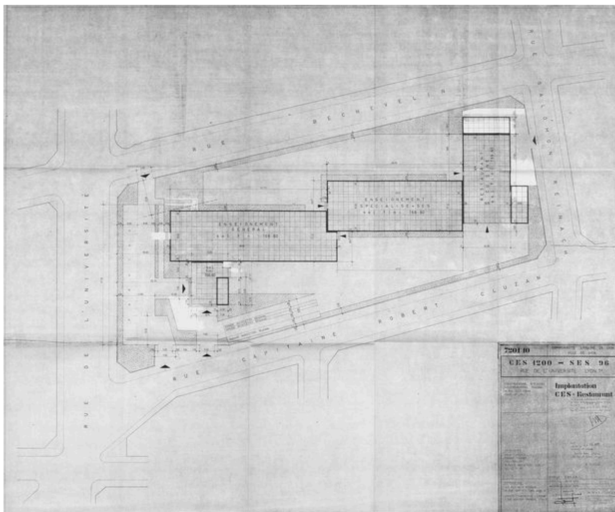
Plan général du rez-de-chaussée (Arch. dép. Rhône, 686 W 189, tirage d'architecte, 1972).
