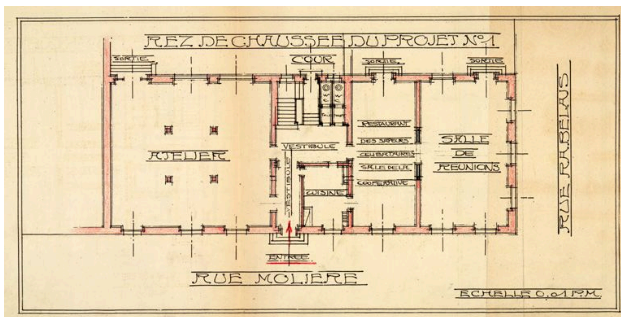
Rez-de-chaussée du projet n°1
