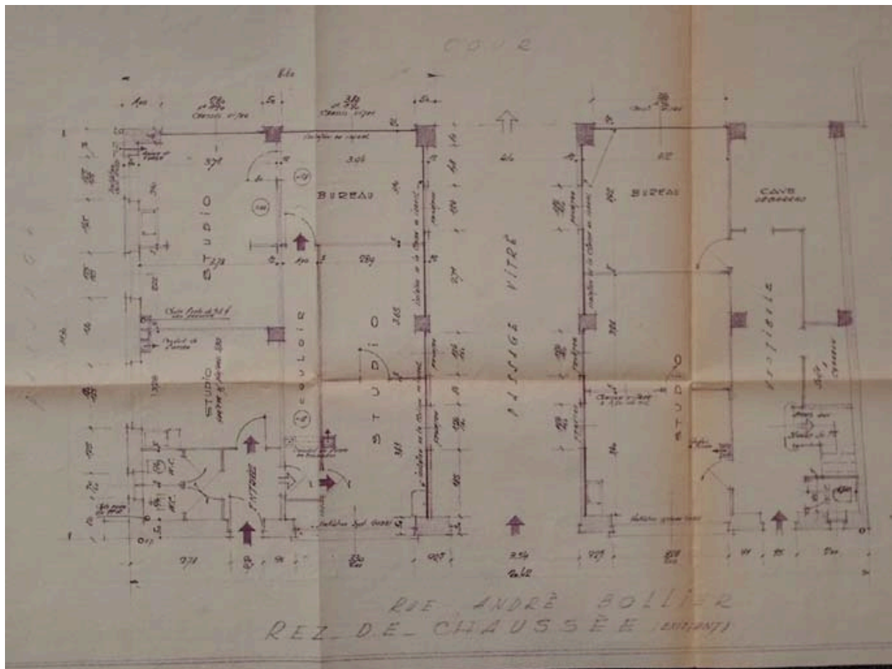
Guignardat ; conciergerie ; plan au sol (1957)
