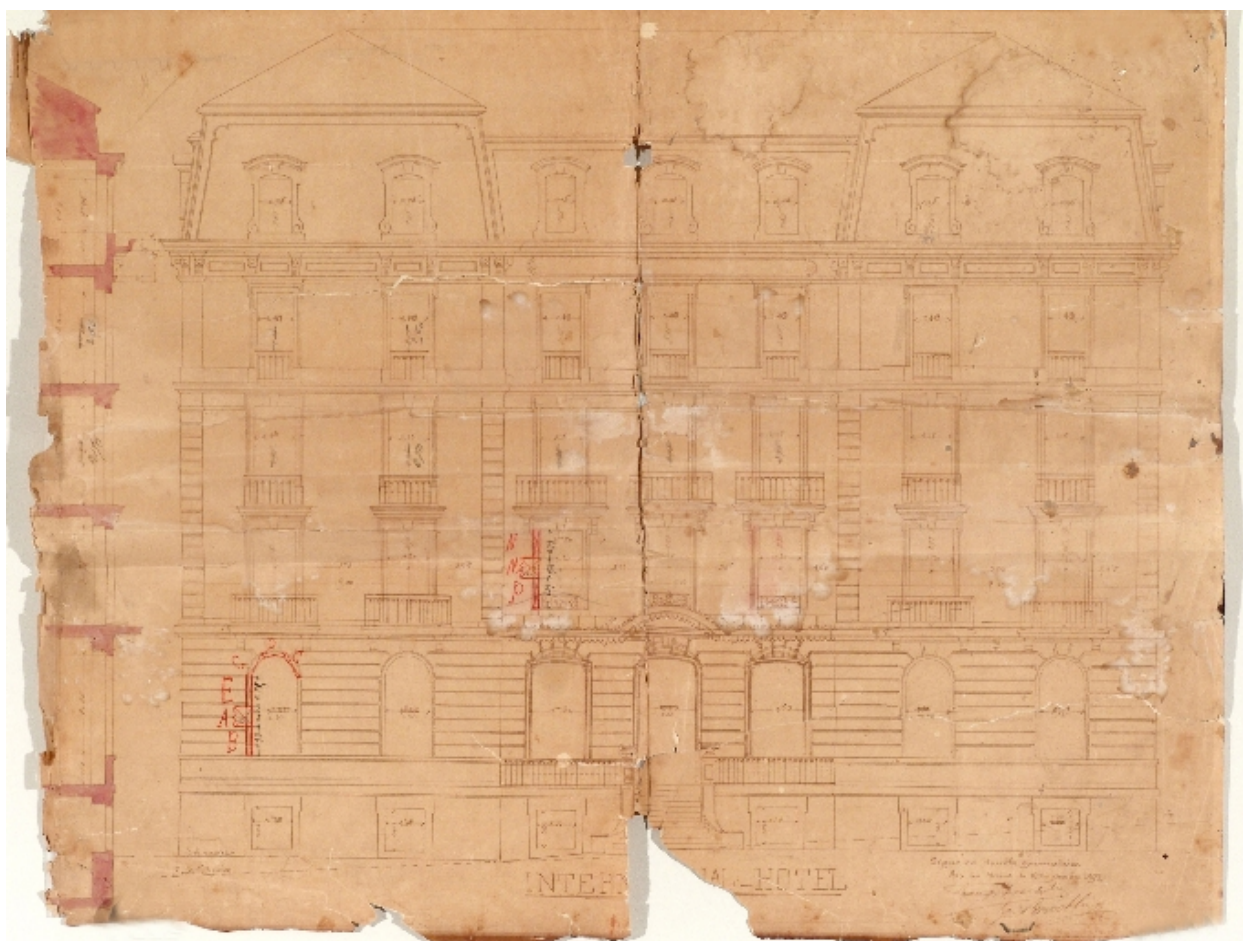
Elévation sud
