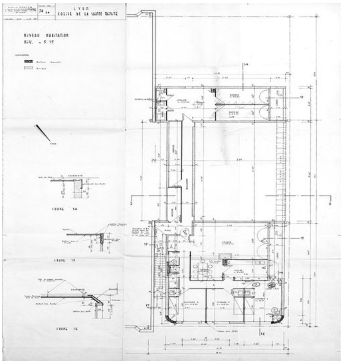
Plan du niveau d'habitation, par P. Genton, février 1961 (A paroissiales Sainte-Trinité, Lyon 8e)
