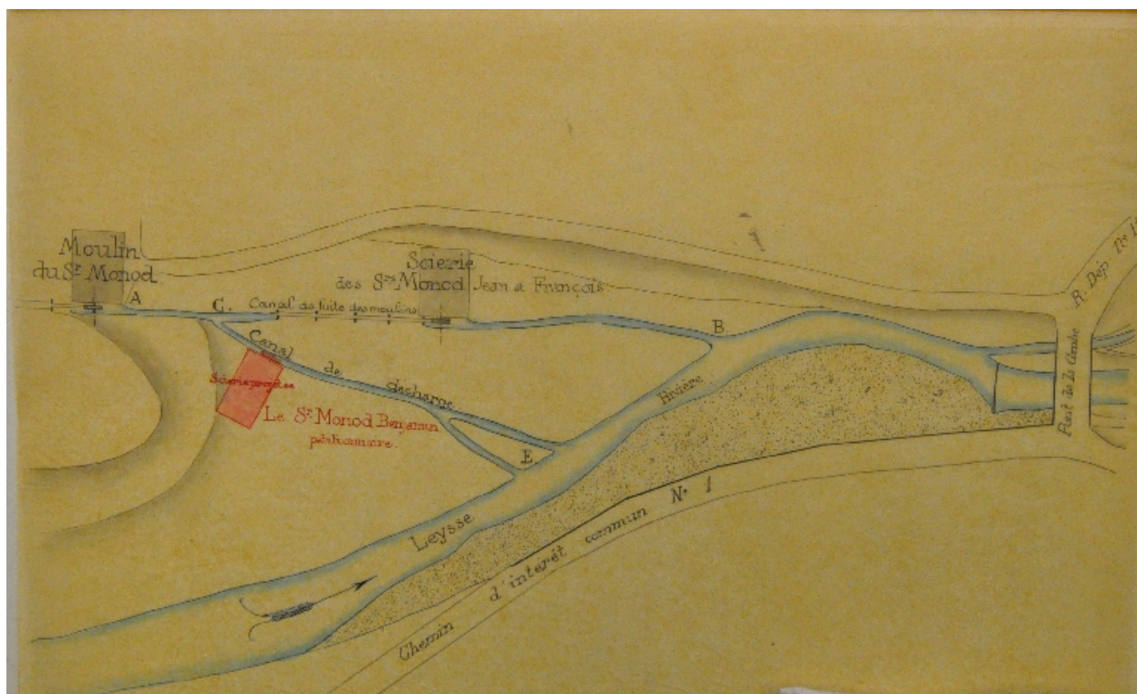
Plan présentant le projet de scierie de Benjamin Monod, 1883
