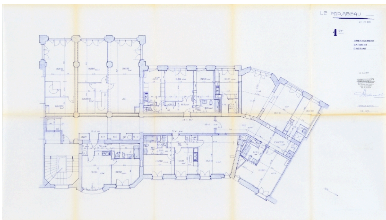
Plan d'aménagement de l'entresol, 1979
