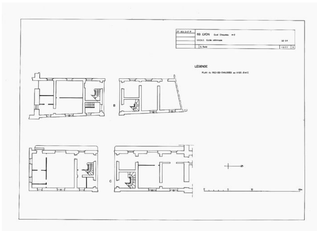
Plan du rez-de-chaussée des bâtiments B et C, relevé Inv. D. Sallé d'après M. Bourdeix, 1941
