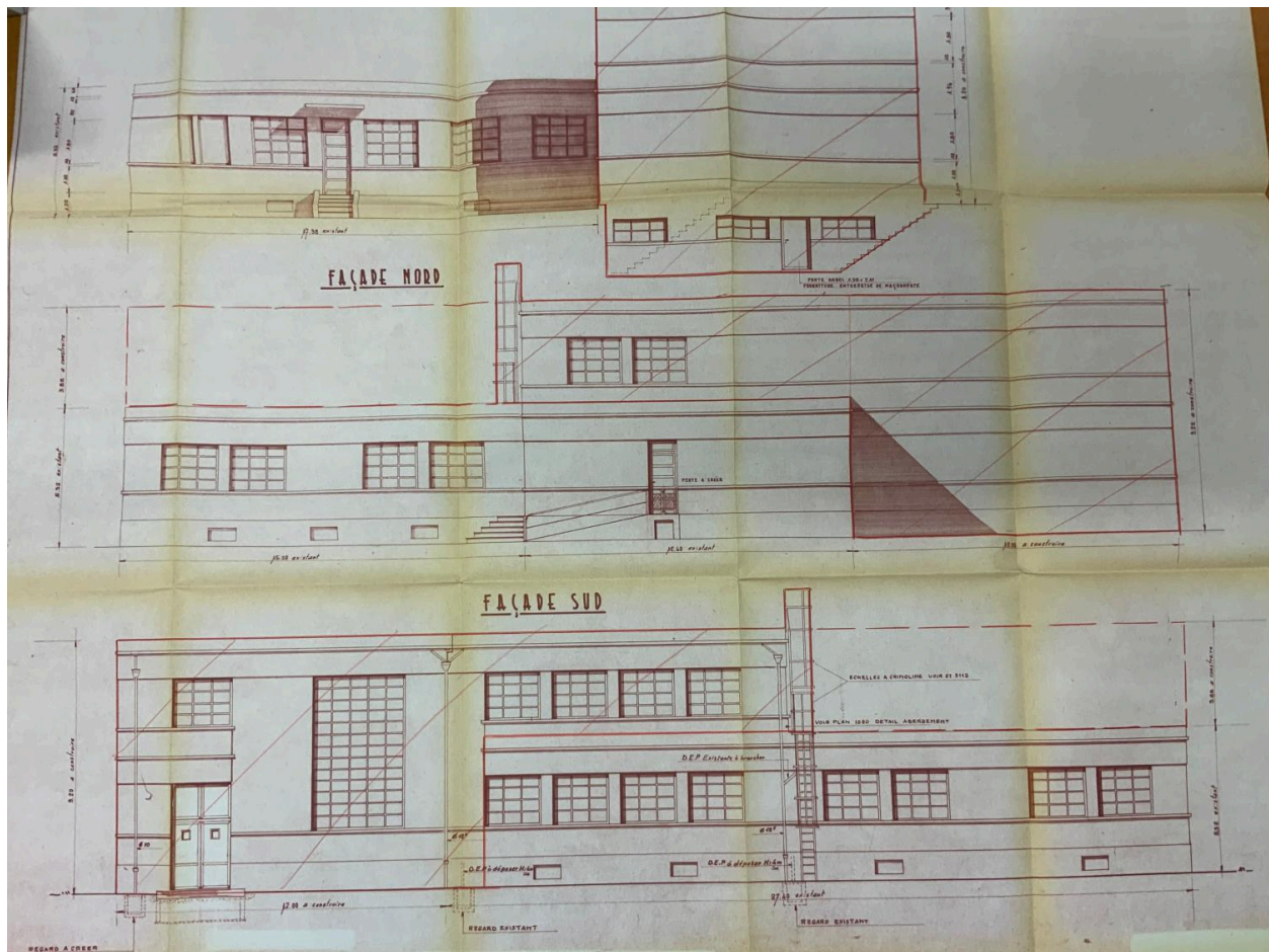
Plan extension des bâtiments de fabrication et ateliers, tracé par J. Denis, 1971 (AC Pierre-Bénite : 203 – 45)
