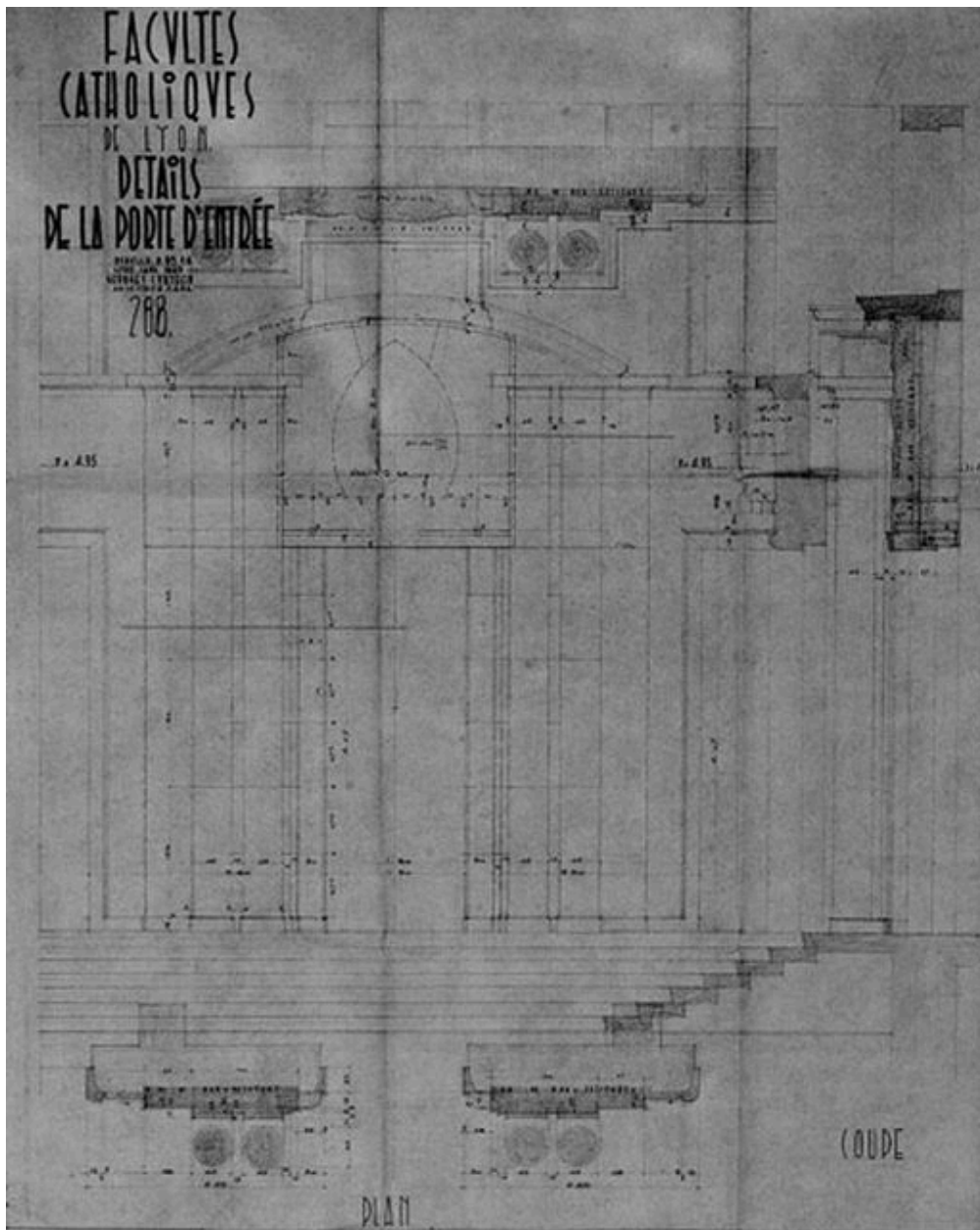
Plan, détail de la porte d'entrée par G. Curtelin, 1943
