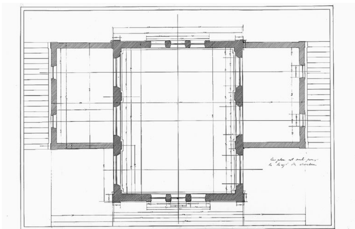
Bâtiment de clinique, plan
