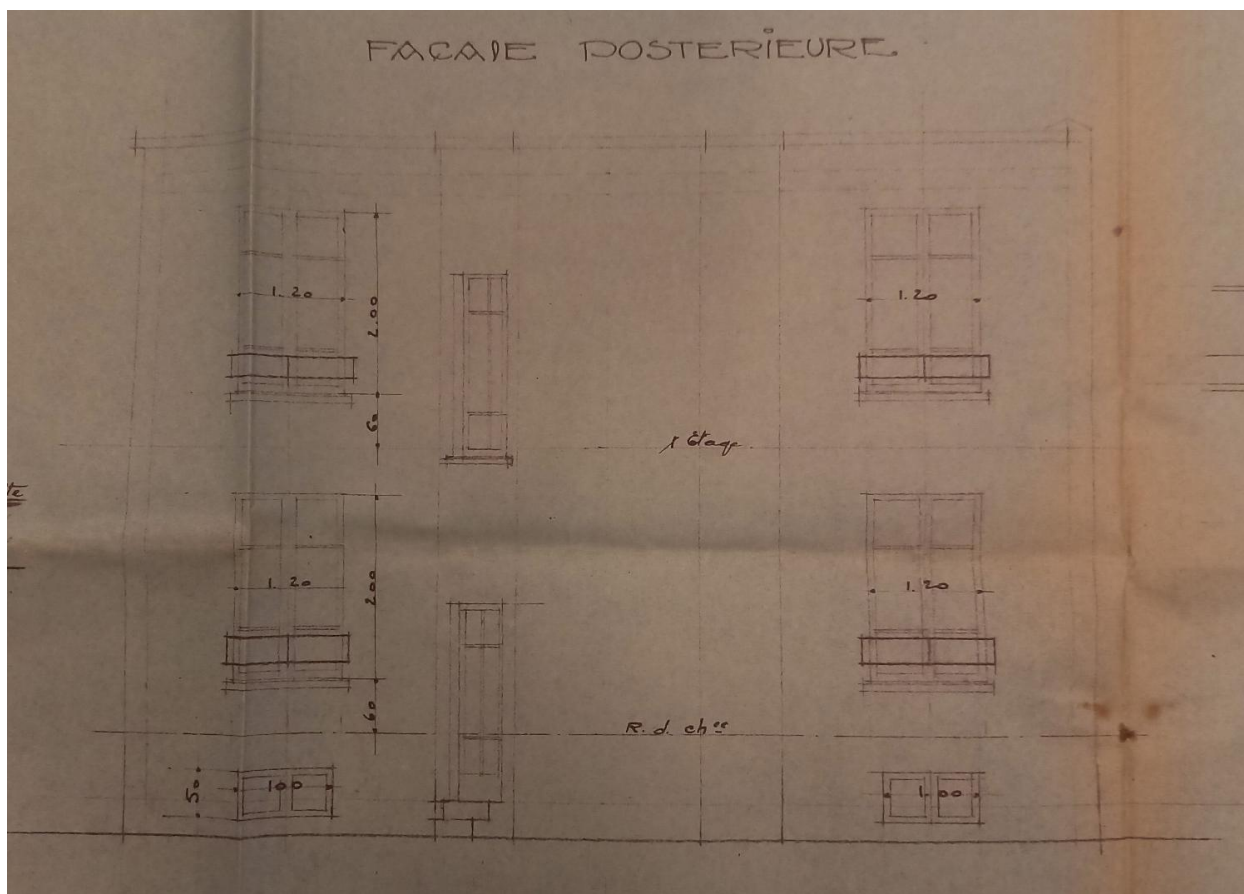
Elévation postérieure
