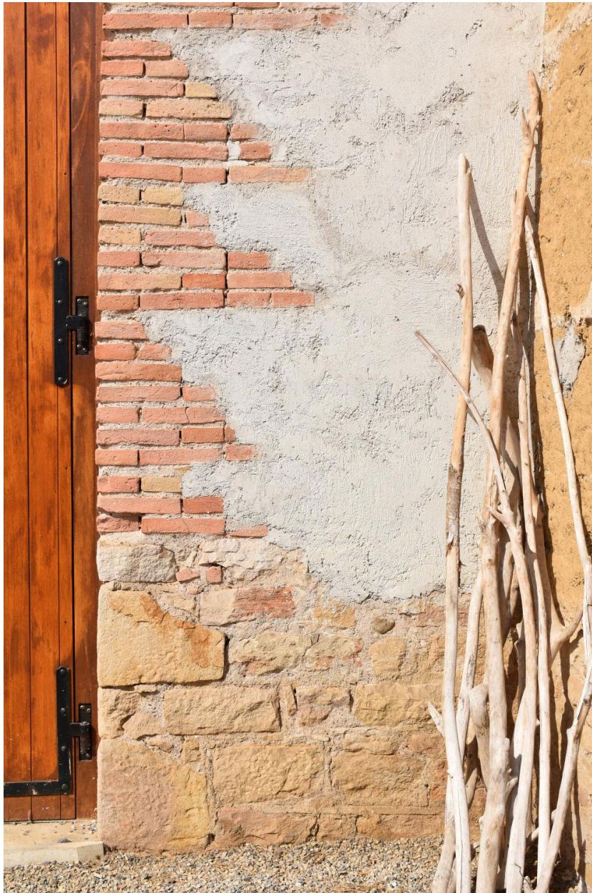
Détail de soubassement et renfort d'angle
