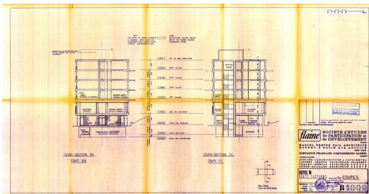
Hôtel B. Coupes transversales. Marcel Breuer architecte, Robert F. Gatje associé, 15 janvier 1962. Modification 9 mars 1962 (AC Arâches-la-Frasse)
