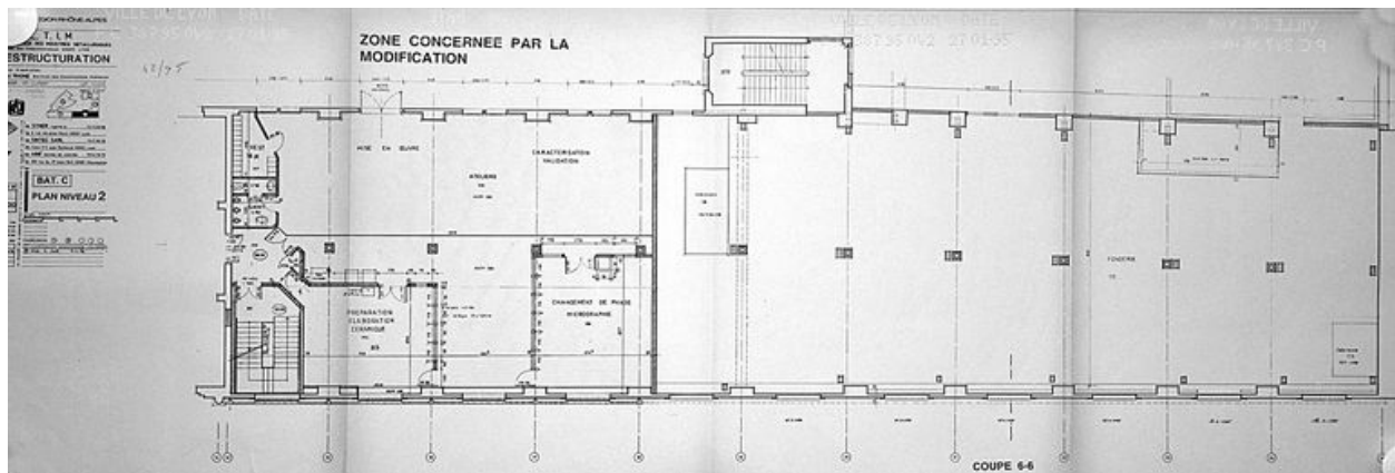
Bâtiment C : plan niveau 2 (Curtelin Ricard), 1995
