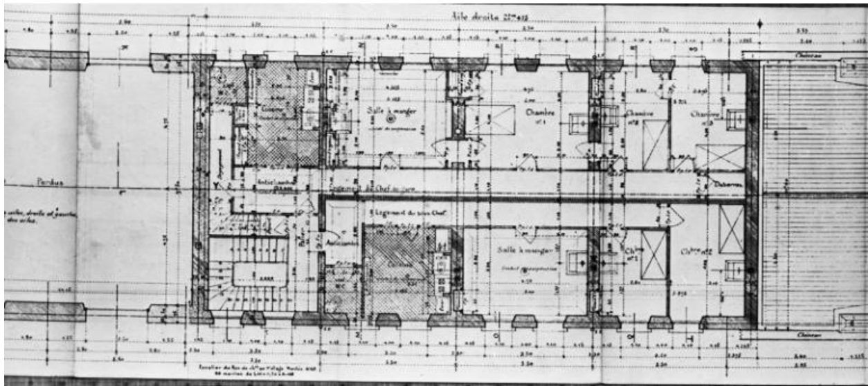
Gare de Châtel-Guyon. Bâtiment des voyageurs. Plan du premier étage.
