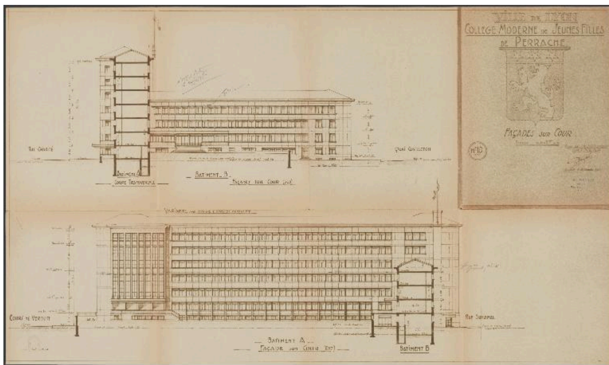
Façades sur cour, par E. Payen, 1954 (AC Lyon, 838 WP 001)
