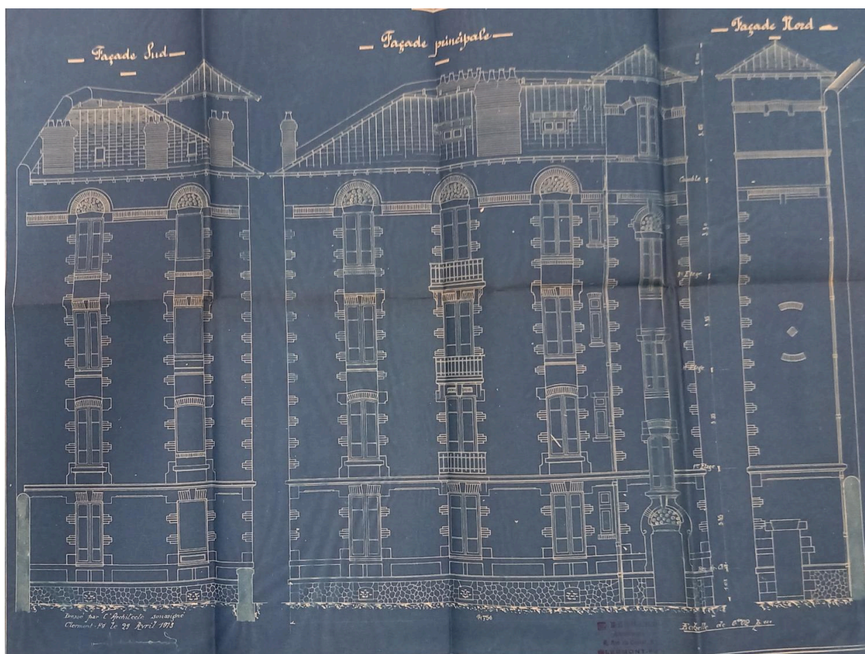
Plan des élévations du 24 avenue d'Italie
