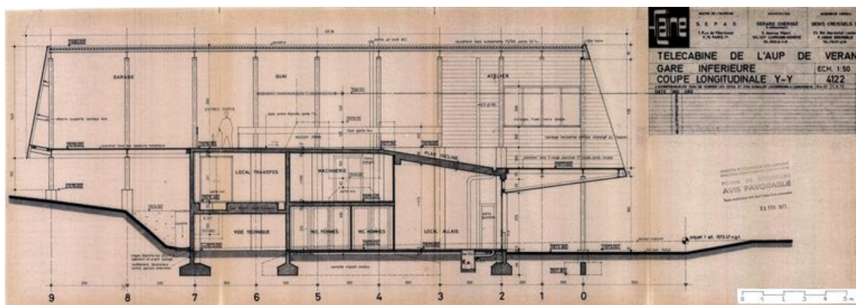
Coupe longitudinale. Gérard Chervaz architecte, Denis Creissels ingénieur conseil, 11 août 1972 (AC Magland)
