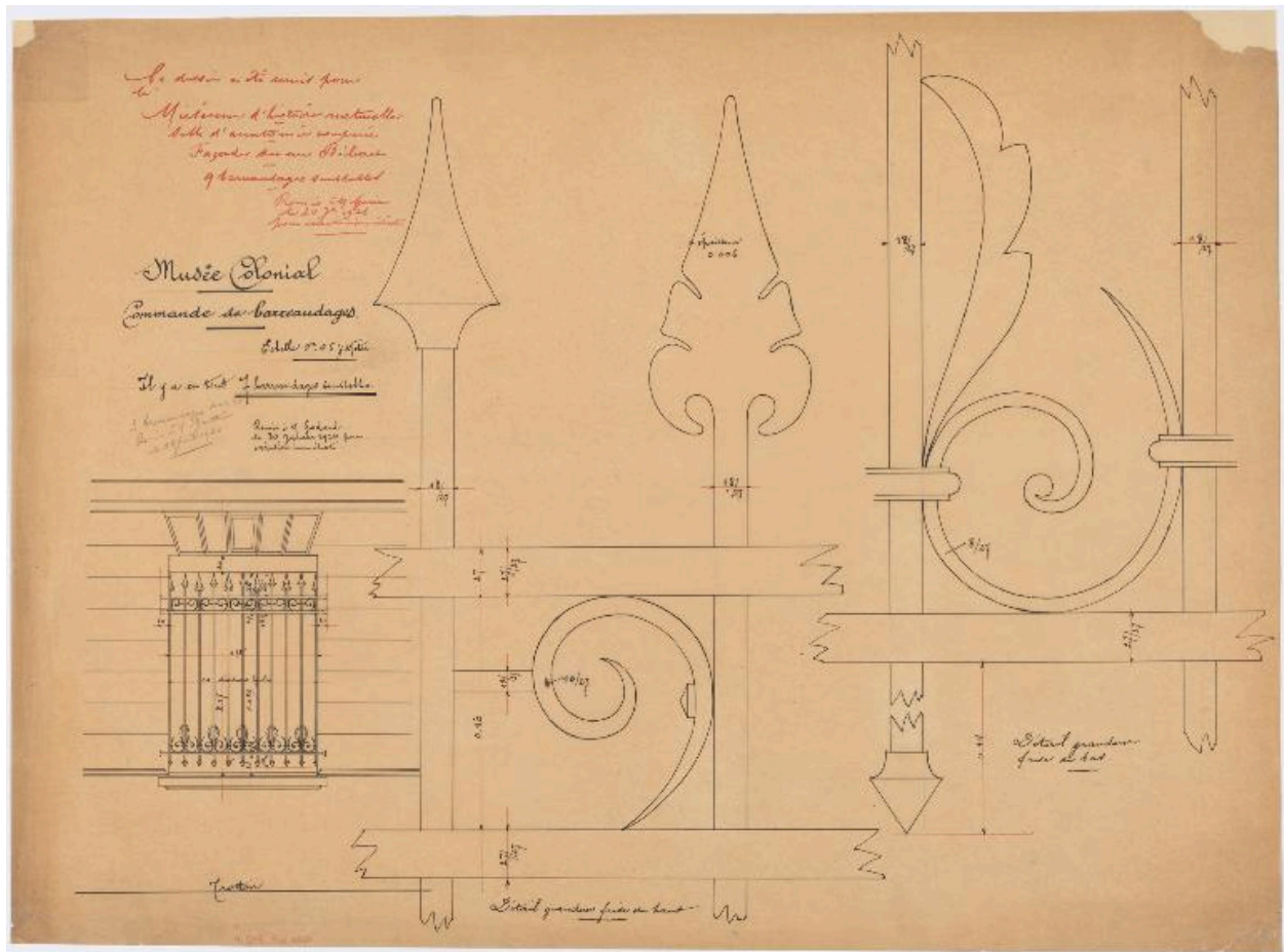
Musée colonial, commande de barreaudages. AC Lyon, 1480 WP 312 P
