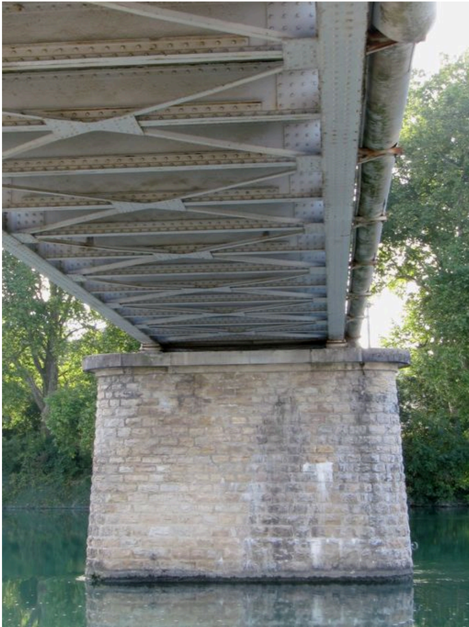
Vue partielle, de dessous, tablier et pile (depuis la rive droite)
