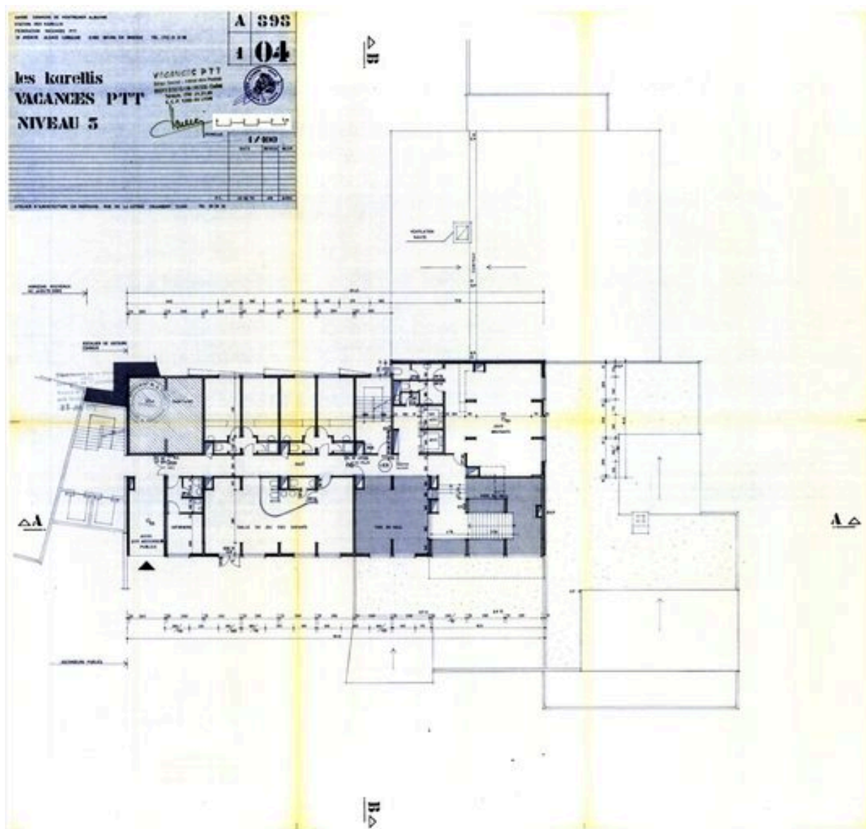
Vacances PTT. Plan niveau 3 / Atelier d'architecture en Montagne, Guy Rey-Millet, 23 mars 1976 (AC Montricher-Albanne)
