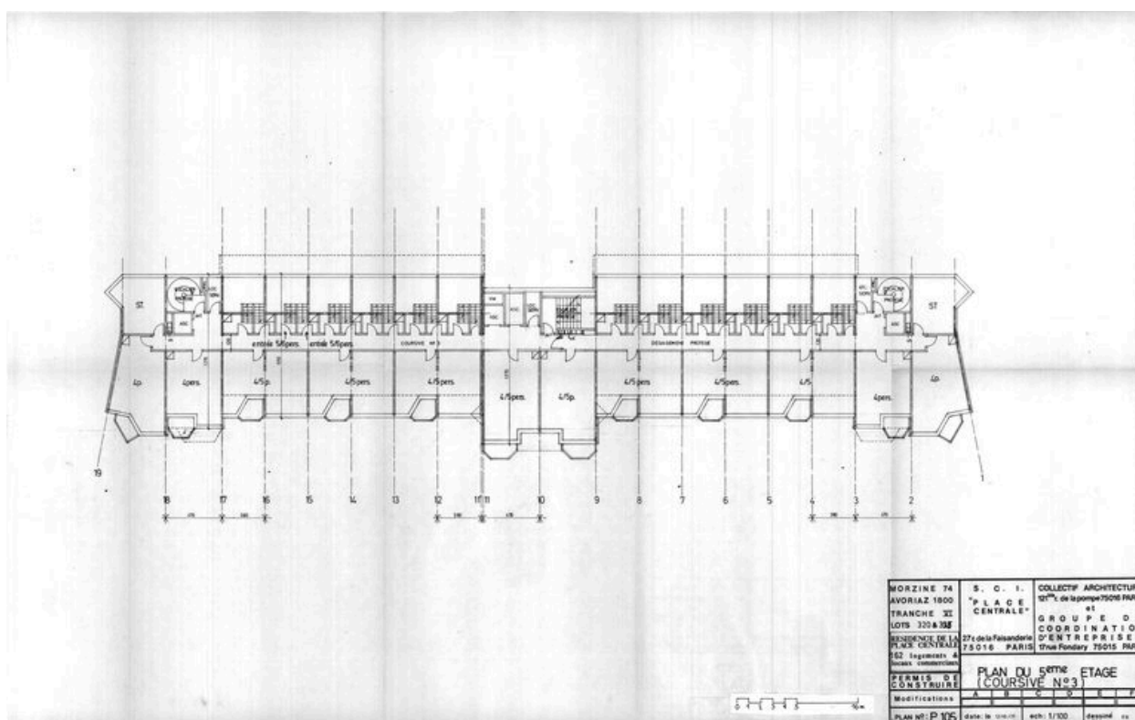
Plan du 5e étage (coursive n° 3) / Collectif architecture et groupe de coordination d'entreprise, 12 octobre 1977 (AC Morzine)
