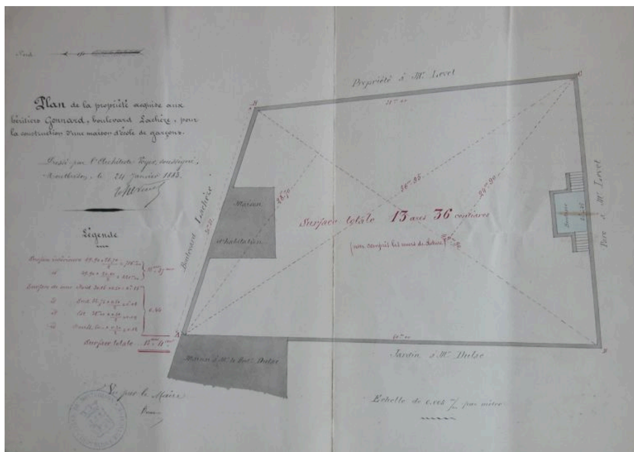
Plan de la propriété à acquies des héritiers Gonnard (AC. Montbrison : série 4W 99). plan 1883 AC Montbrison. 4W 99
