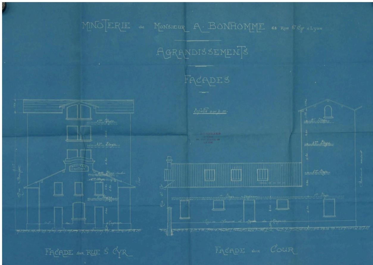
Plan de la minoterie Bonhomme à Vaise 1913 (ACL 314W514-822)
