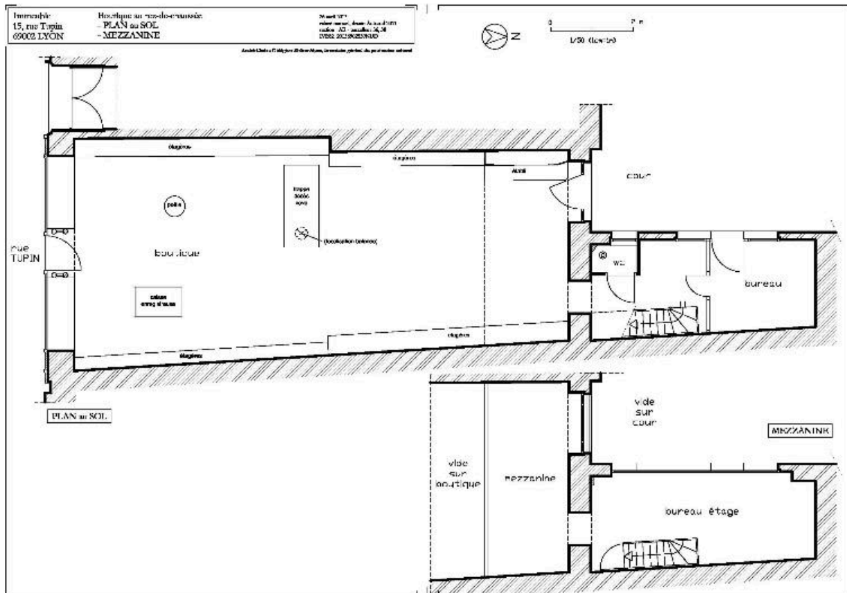
Boutique : plan du rez-de-chaussée et plan de la mezzanine
