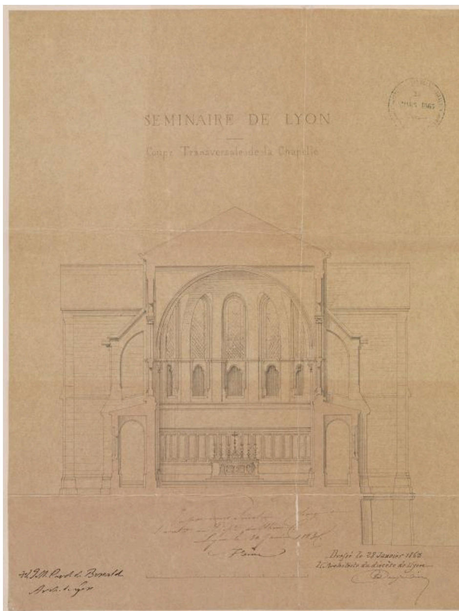
Coupe transversale de la chapelle, par Tony Desjardins, 1863 (AD Rhône, 3 V 29/3)
