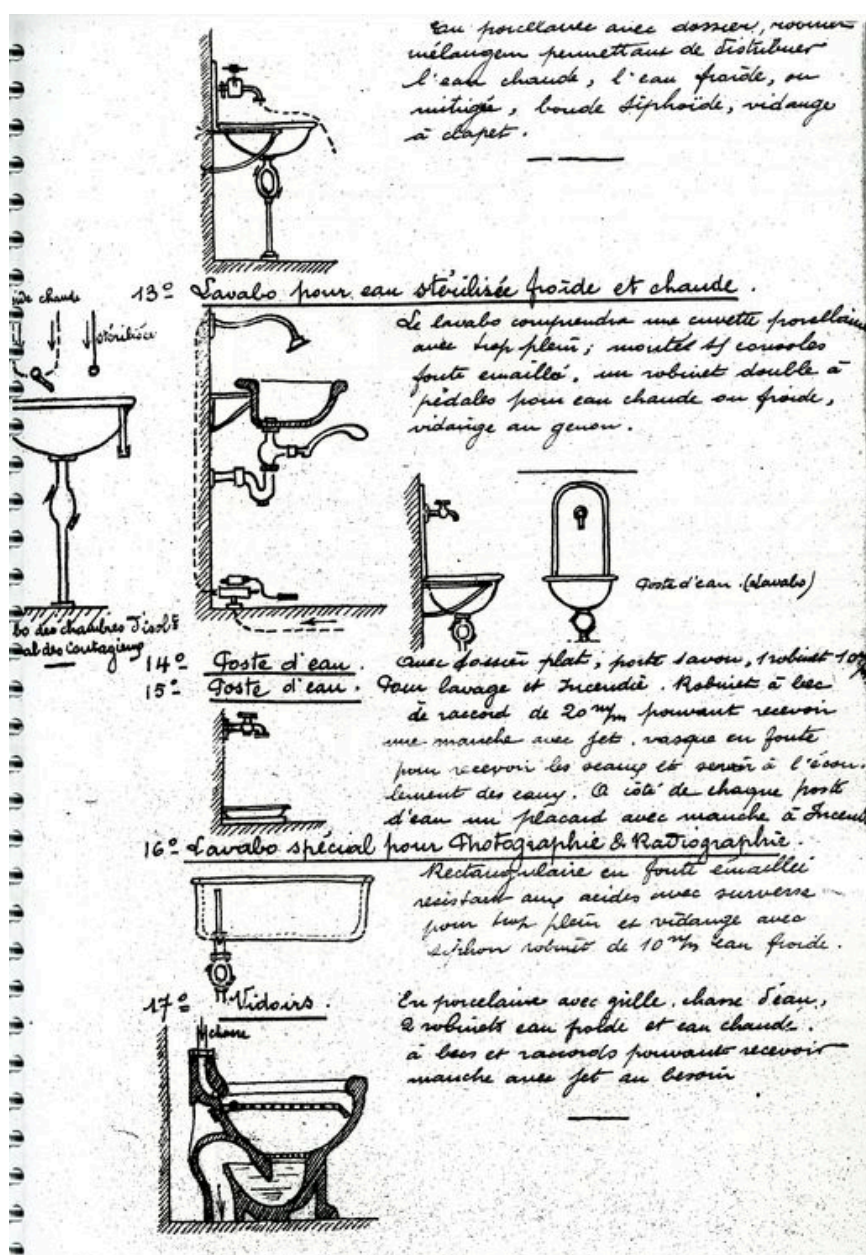
Dessin des équipements sanitaires / Tony Garnier, 30 novembre 1910
