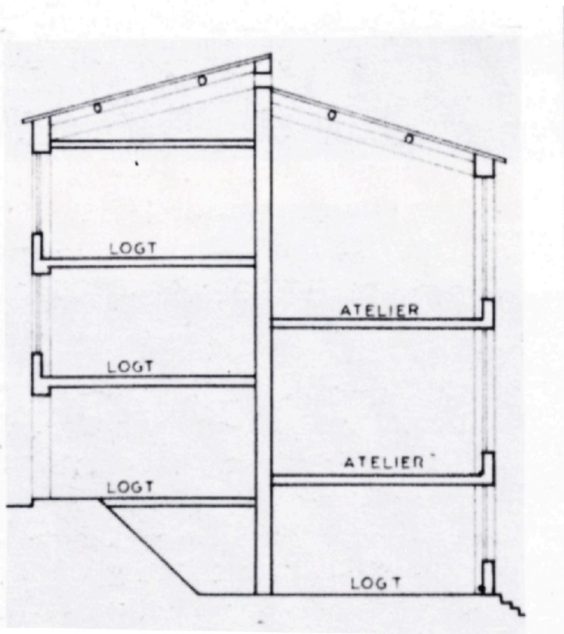
Coupe d'un immeuble-atelier de passementier
