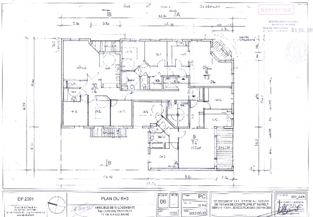
Plan du troisième étage
